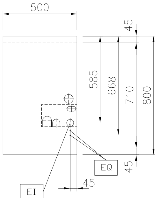
Boven aanzicht
